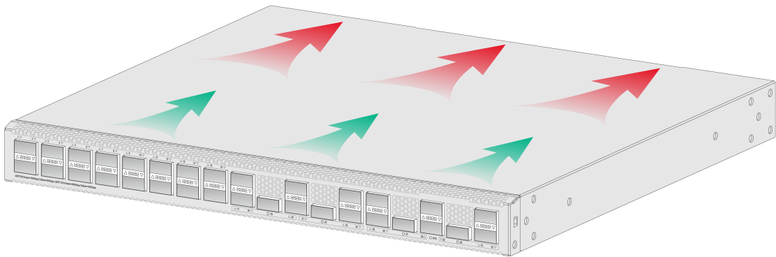
图5-2 可插拔风扇机型散热空气流向示意图（以安装为 LSPM1FANSB1-Z 例）
