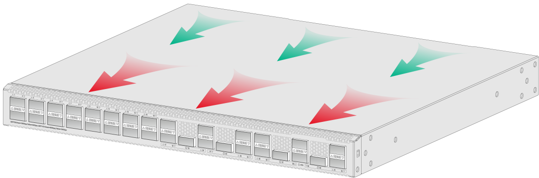
图5-1 可插拔风扇机型散热空气流向示意图（以安装 LSPM1FANSA1-Z 为例）
