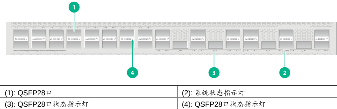
图2-1 S9600XP-32H-G 前面板示意图
