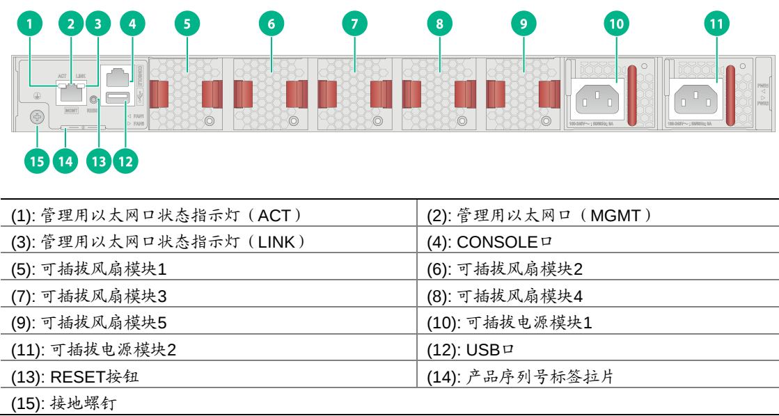
图2-2 S9600XP-32H-G 后面板示意图
